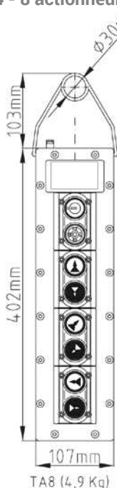
Boîte à boutons simple 4 - 8 actionneurs
