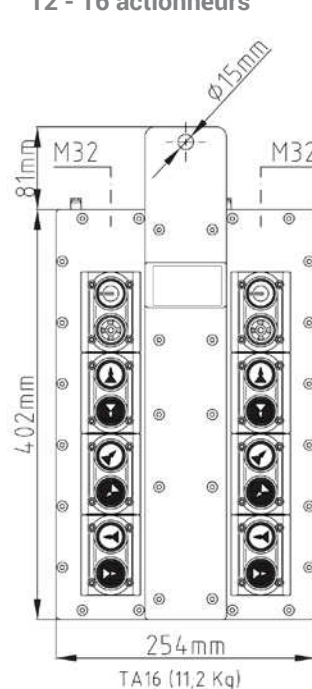
Boîte à boutons double 12 - 16 actionneurs
